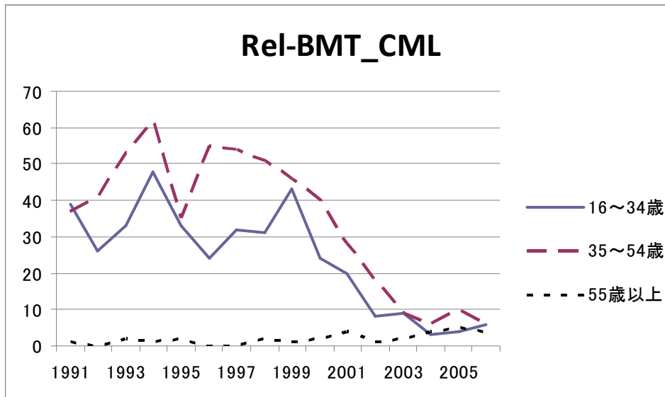
図 11.3 CML
