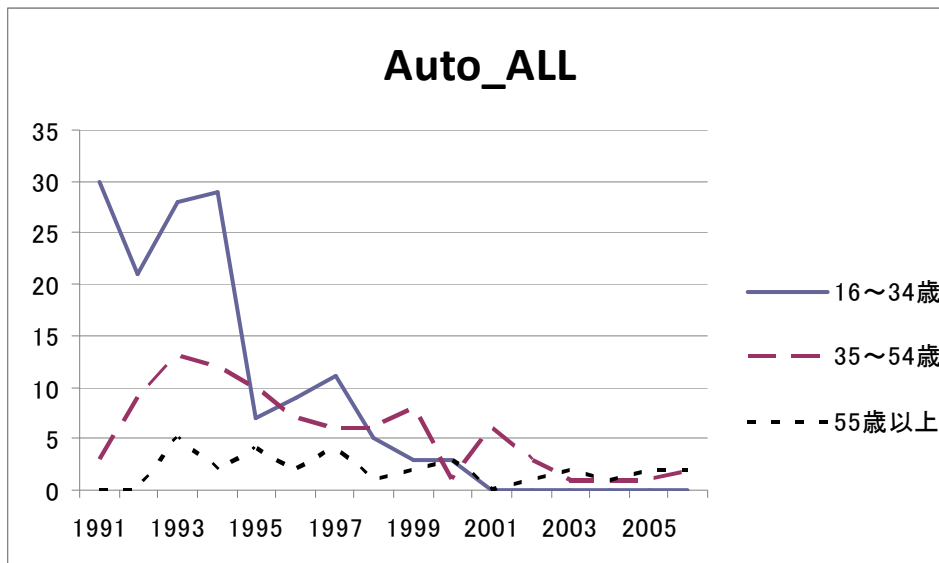
図 11.2 ALL
